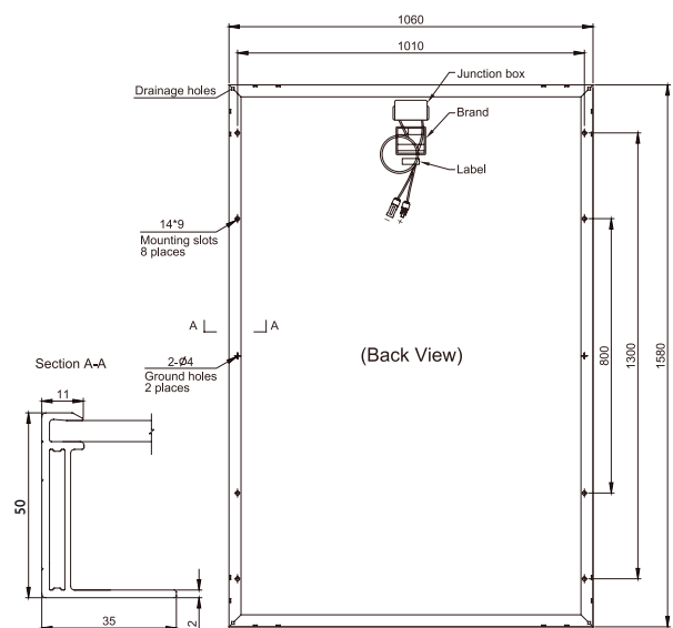
Module Diagram (measures: mm)
