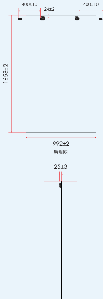
组件尺寸 (单位: mm)
