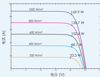
组件的I-V曲线 (170W)
