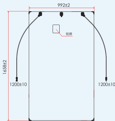
后视图 (横装)
