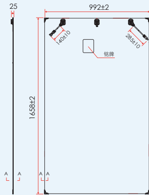
后视图 (竖装)
