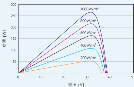
组件的P-V曲线 (265W)
