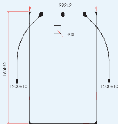
后视图 (横装)
