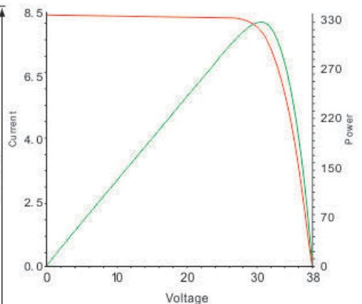
IV测试曲线
