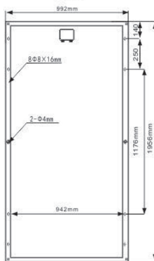
尺寸图
