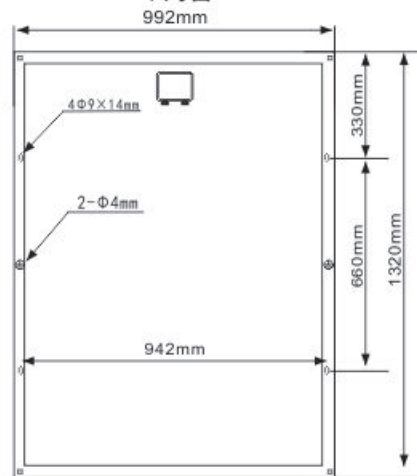
尺寸图
