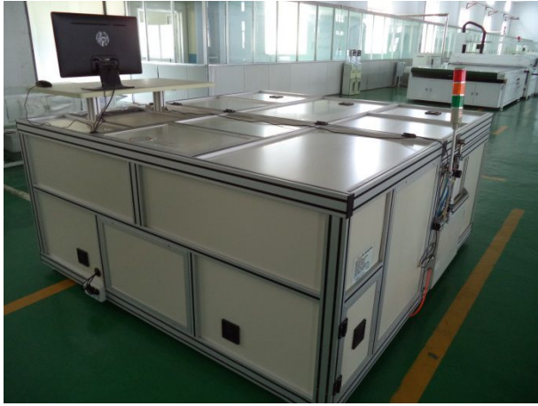
EL Tester
