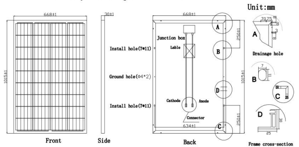
110W Poly solar panel (1015*668*30)
