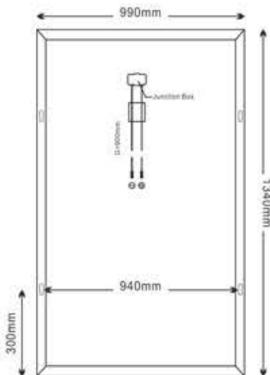
Module Diagram
