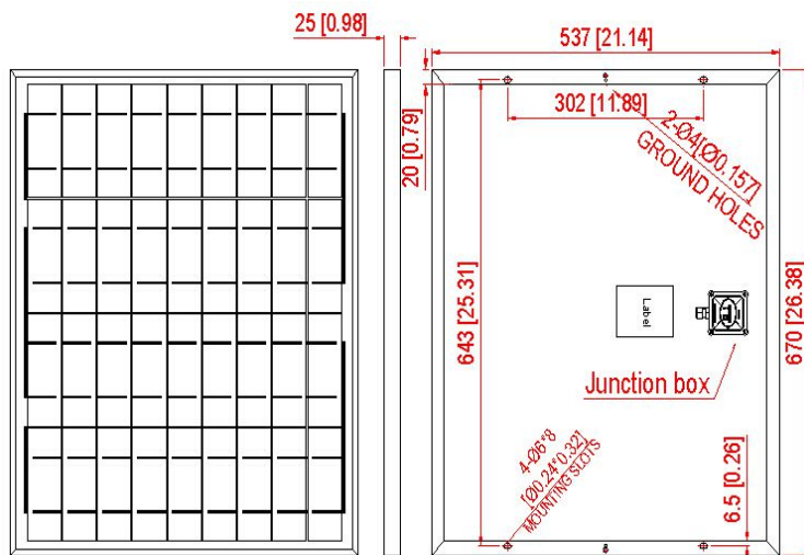
Module Diagram
