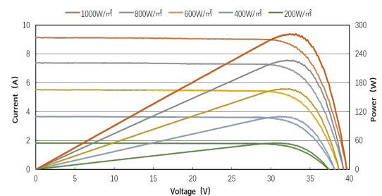
I-V & P-V curve AE DGM6-60
