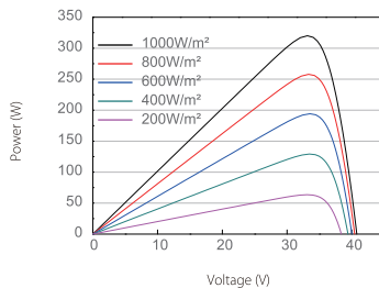
Power-Voltage Curve(AOX-60MS-345W)
