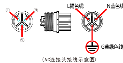
(AC连接头接线示意图)
