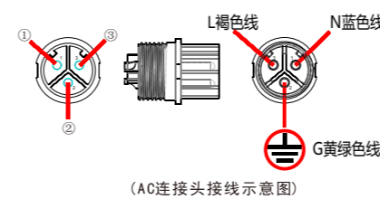
(AC连接头接线示意图)
