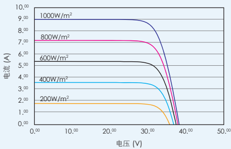
组件的I-V曲线 (260W)
