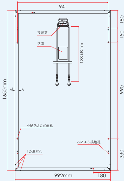
(后视图)
