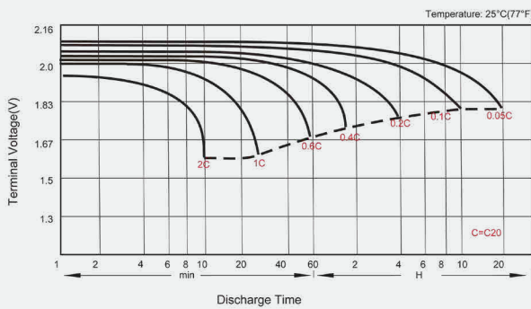
放电曲线 Discharge Characteristics
