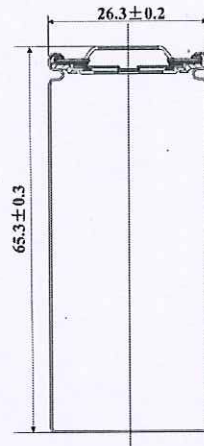
图 1 电芯外观尺寸
