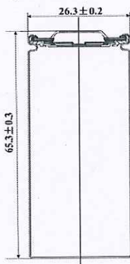
图 1 电芯外观尺寸
