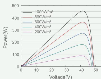
Power-Voltage Curve(SP455M-72H)
