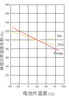
Isc、Voc、Pmax 的温度曲线
