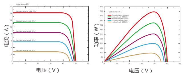
电流电压及功率电压曲线(SKT550M10)
