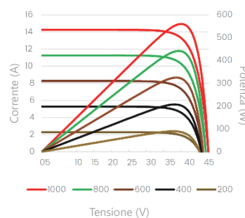
Curva corrente-tensione e potenza-tensione (560W)
