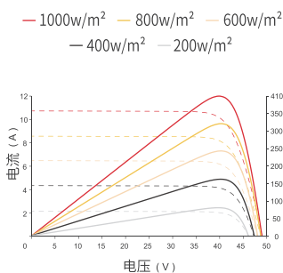
电流 - 电压 & 功率 - 电压曲线图 (415W)
