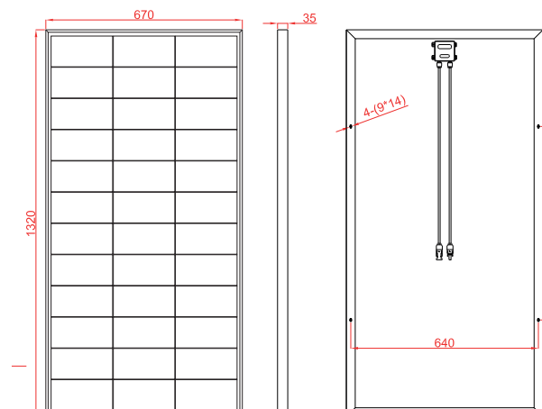
Dimensiones - Dimensions ESF-165MD
