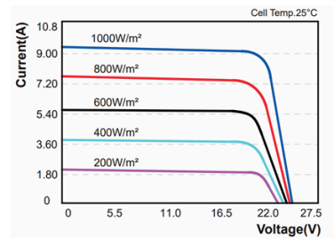
Resultado de la medición de potencia PVPM Result of PVPM Power Measurement
