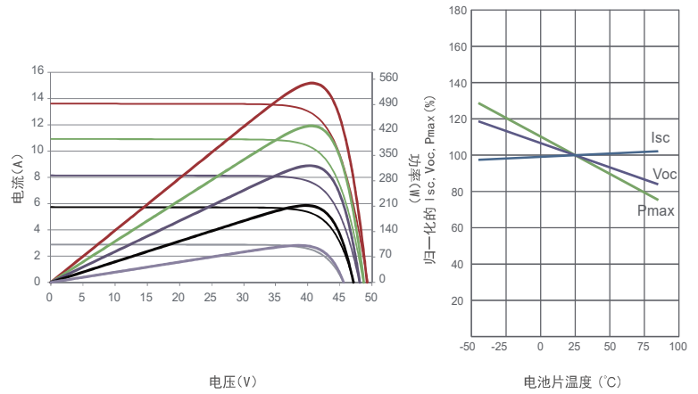
电流电压及功率电压曲线(550W)
