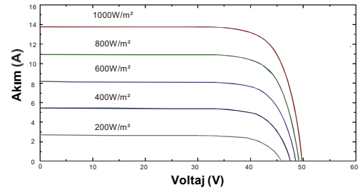
Akım - Voltaj Grafiği (ECT 540-144PMB10)
