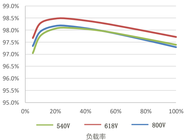
效率曲线
