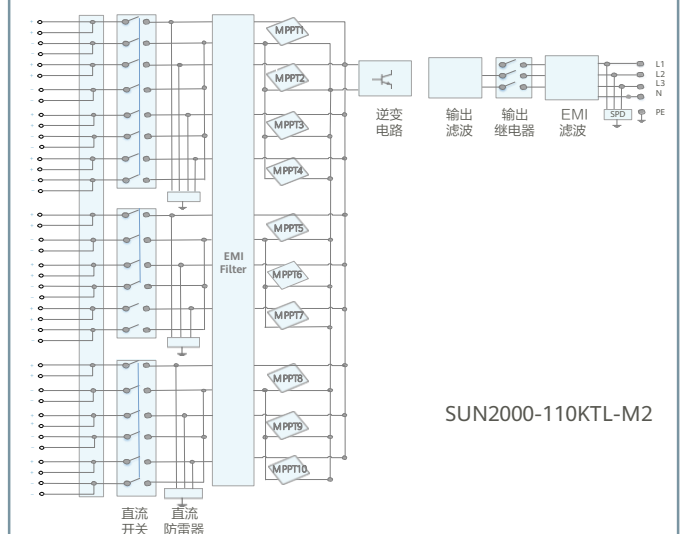
电路框图
