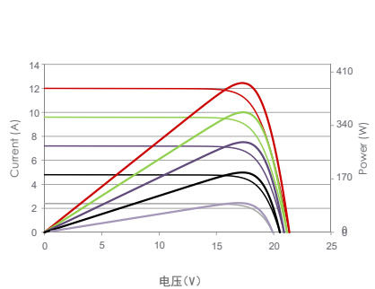
电流电压及功率电压曲线
