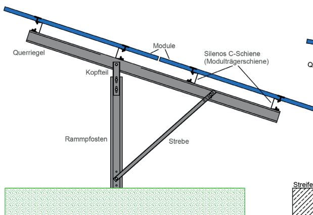
Bsp. 1-Pfosten-Rammsystem
