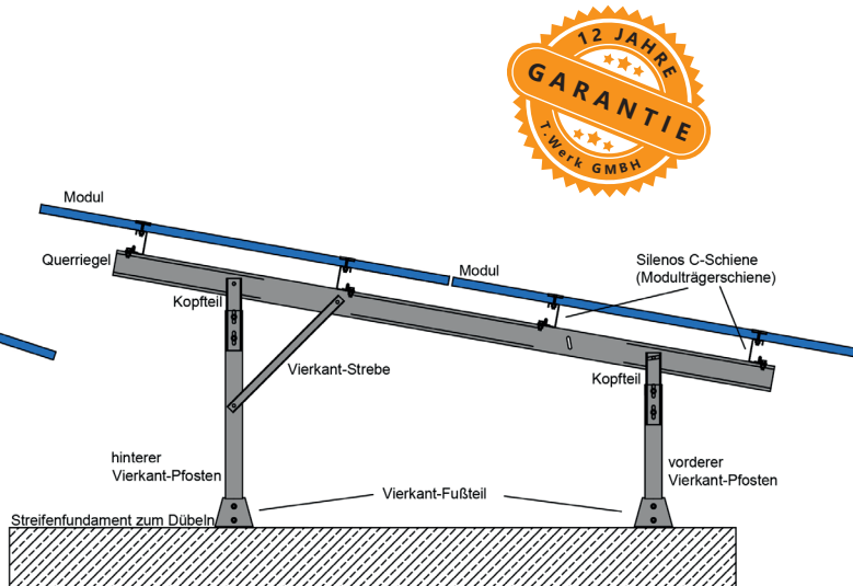
Bsp. 2-Pfosten-System zum Aufdübeln auf Streifenfundamente
