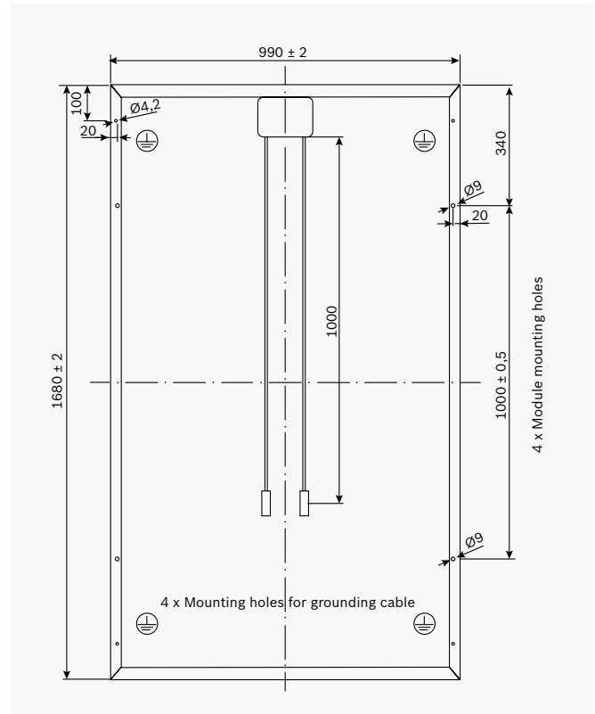
Abbildung 4: Rückseite c-Si M 60, Hersteller 13
