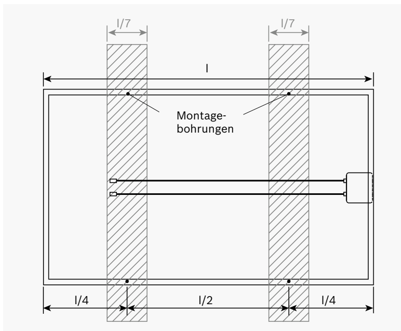
Abbildung 2: Befestigungsbereich horizontal
