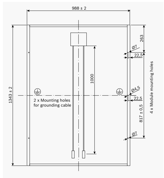
Abbildung 6: Rückseite c-Si M 48 und P 48, Hersteller 11
