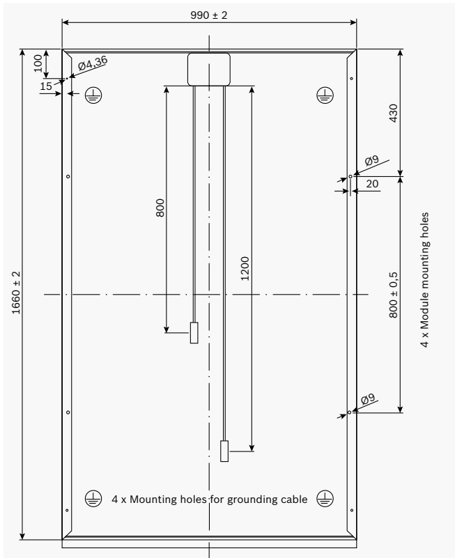
Abbildung 3: Rückseite c-Si M 60 und M 60 S, Hersteller 14, 17 und 23
