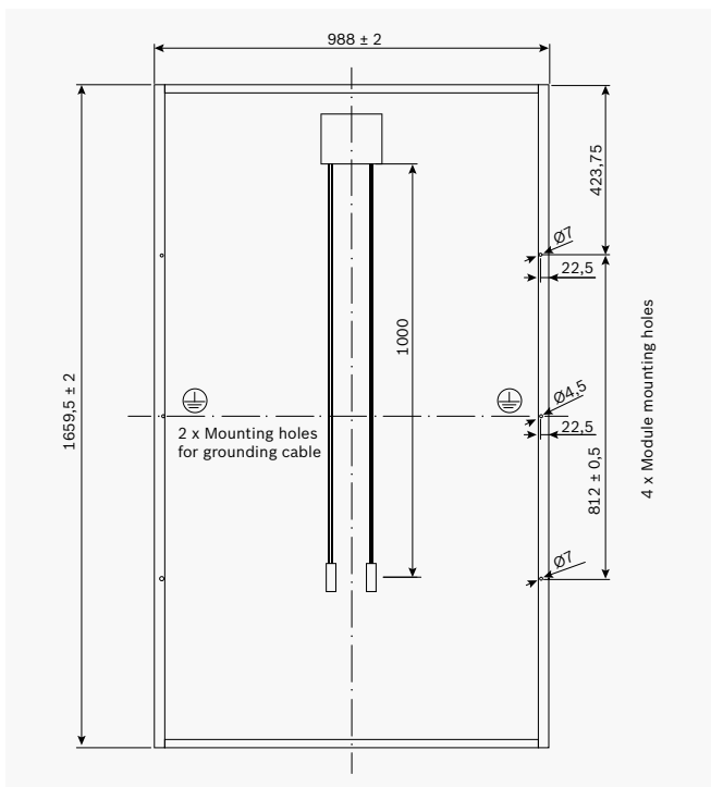
Abbildung 5: Rückseite c-Si M 60 und P 60, Hersteller 11
