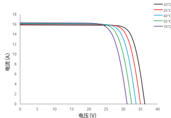
电流-电压曲线 SSA-48HDB-445N
