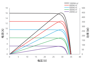
电流/功率-电压曲线 SSA-48HDB-445N
