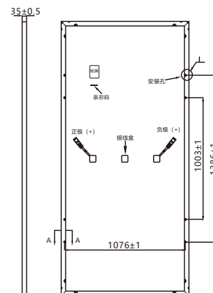
组件尺寸 Dimension
