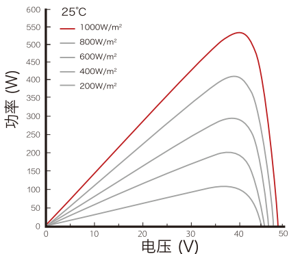
功率—电压曲线 OLV-535-72M-HEAH
