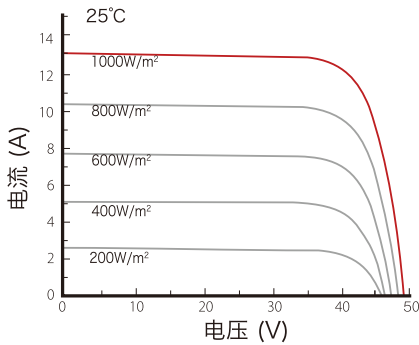
电流—电压曲线 OLV-535-72M-HEAH
