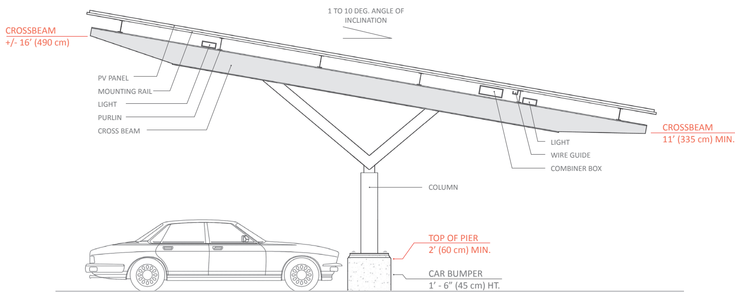
TYP. END ELEVATION
