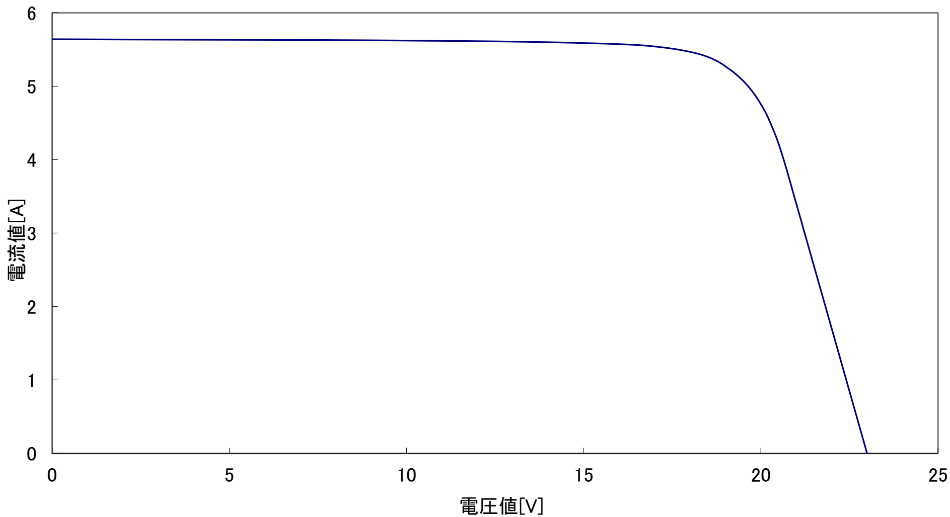
GN100R 出力特性図 @1000W/m 2 AM1.5 25°C
