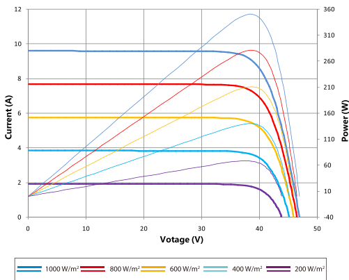
电流-电压 & 功率-电压曲线图 (345W)
