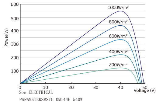
Power--Voltage
