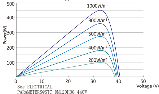
Power--Voltage
