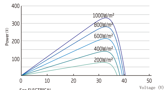
Power--Voltage
