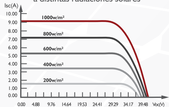
Curva I-V de módulo SAYA-P305-60 a distintas radiaciones solares
