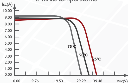
Curva I-V de módulo SAYA-P305-60 a varias temperaturas
