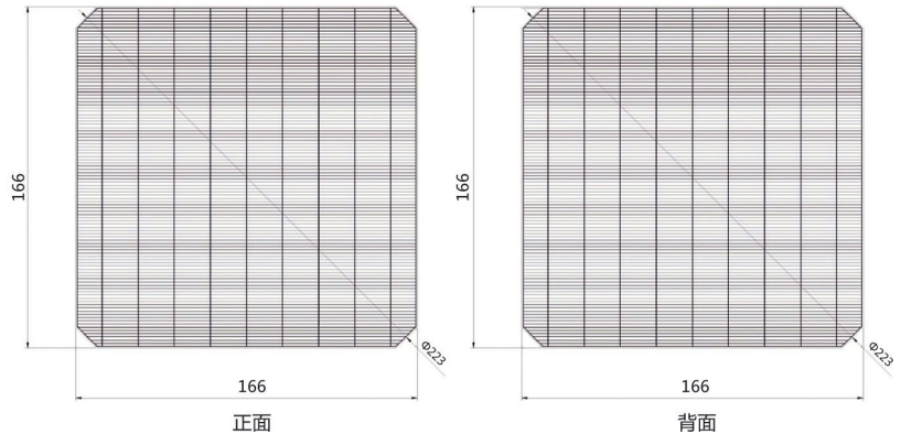
尺寸图 (mm)
