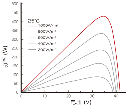
功率-电压曲线 OLV-445-60M-DEAH
