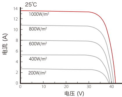
电流-电压曲线 OLV-445-60M-DEAH
