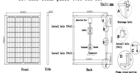
85W Mono solar panel (780*668*30)
