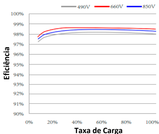
Curva de Eficiência do Inversor
