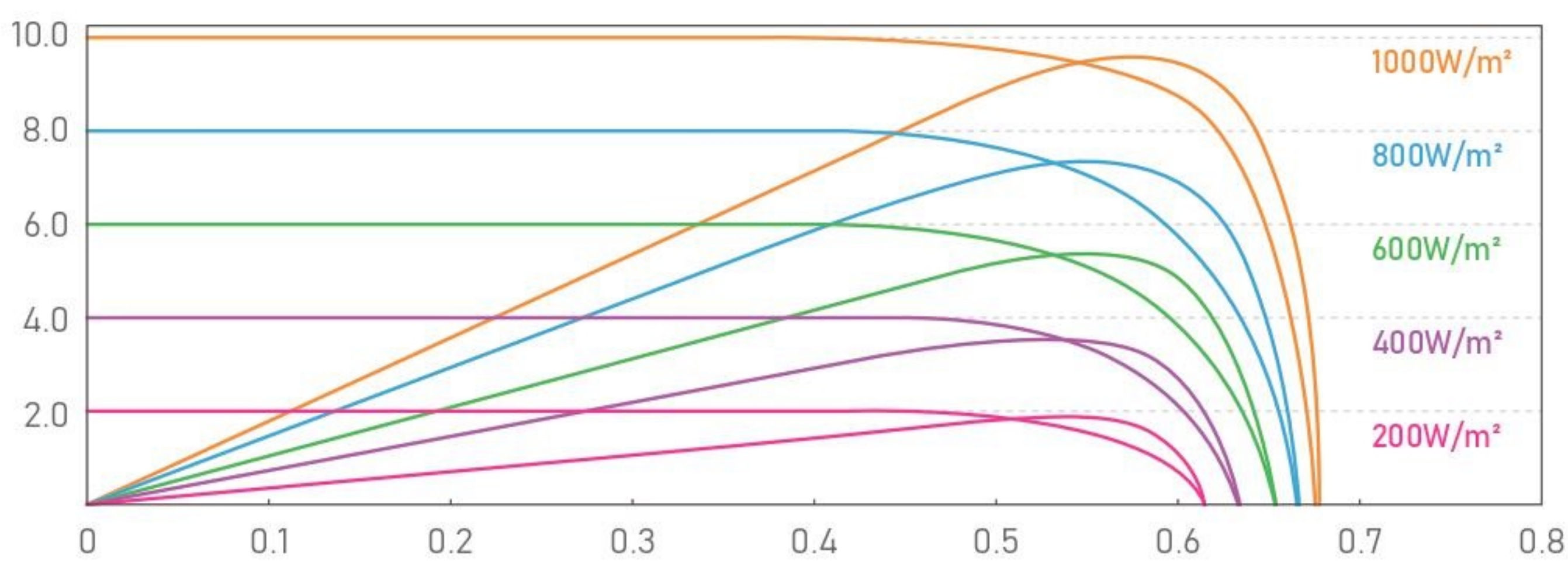
IV 曲线
