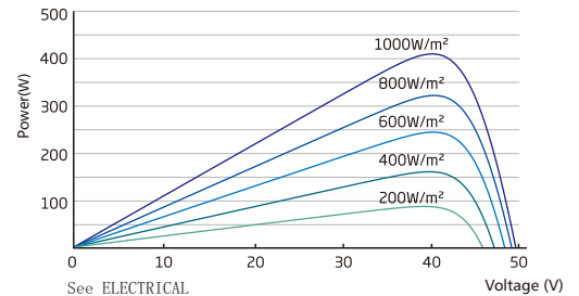
Power--Voltage
